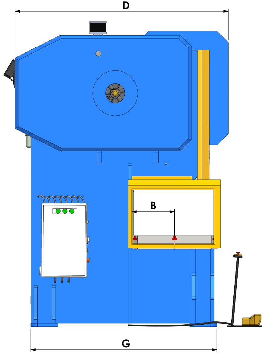
Yan Görünüş Side View
