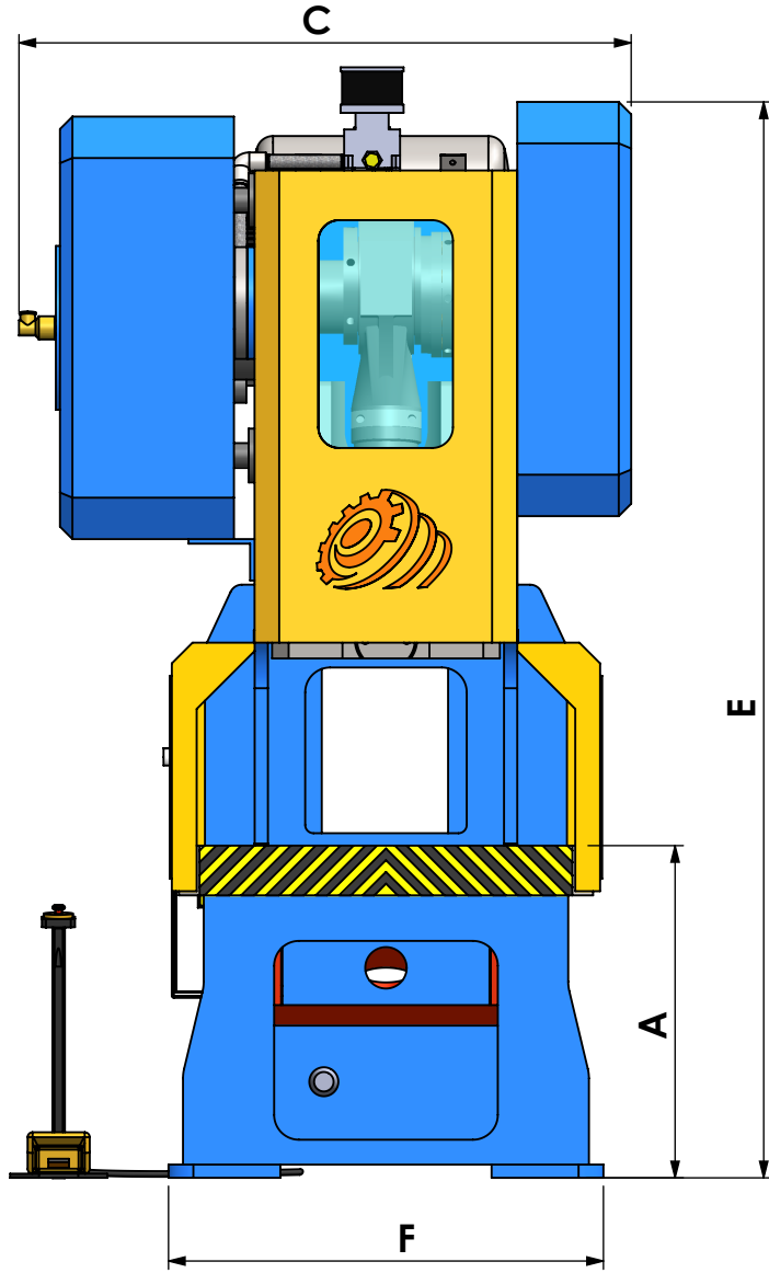
Ön Görünüş Front View
